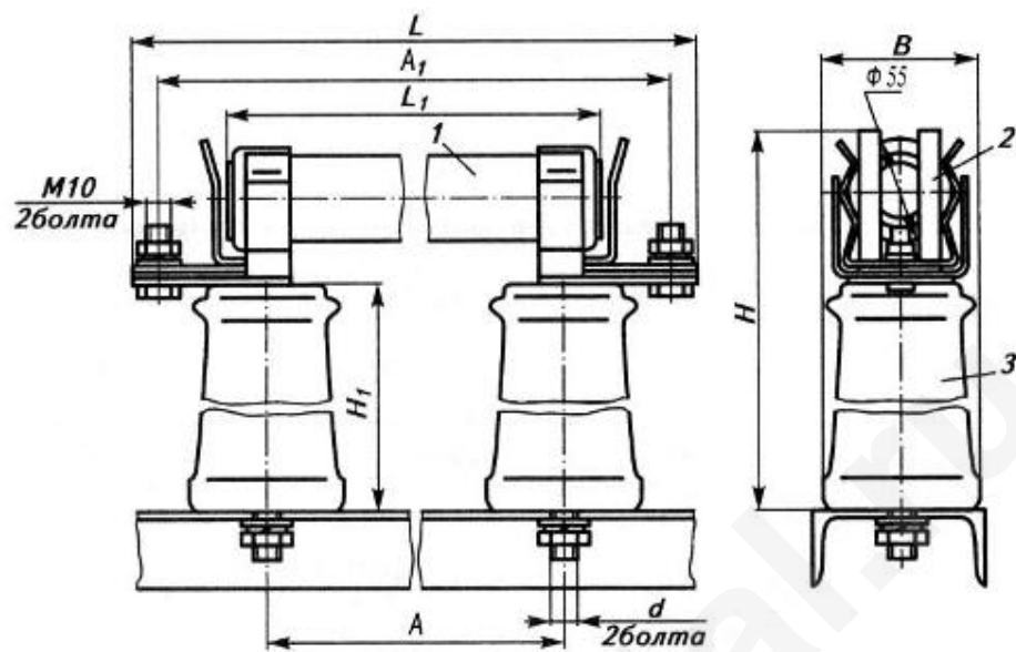
Рис.1 Габаритные, установочные и присоединительные размеры предохранителей серии ПКН001 (исполнение УЗ )
